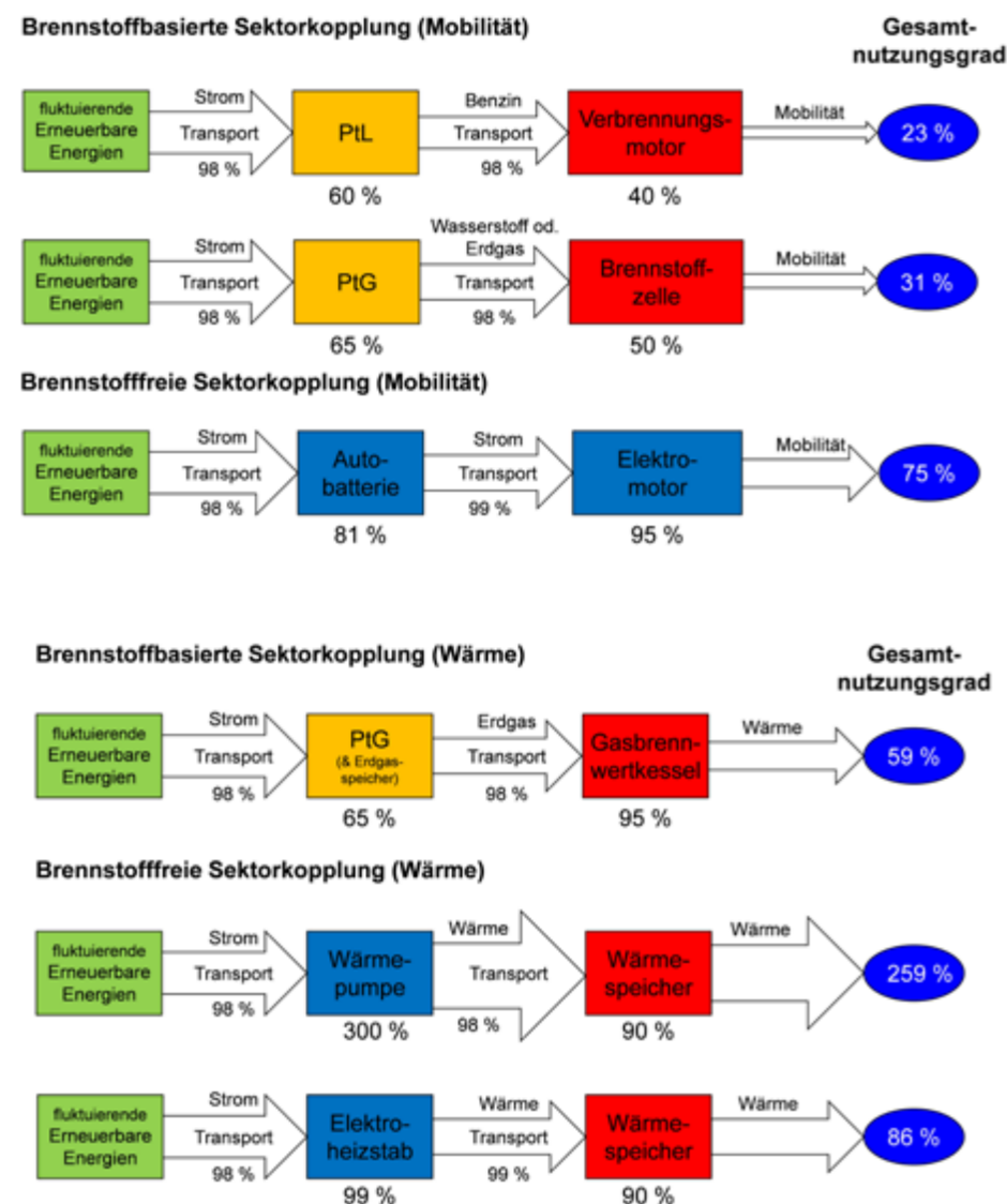
Abb. 2: Energetische Wirkungsgradketten im Wärme- und Verkehrssektor (exemplarische Auswahl mit üblichen Werten z.B. Appellrath et al. 2012). Je nach Systemgrenze, ergänzenden Annahmen und Datenauswahl gelangen diverse Studien stets zu unterschiedlichen Werten für Wirkungsgrade. Doch selbst bei Anlegen von Spannweiten oder das Abstellen auf die Top-Runner jeder Technologie dürfte für die Verwendungsregeln im Wesentlichen dieselbe Reihenfolge resultieren.
